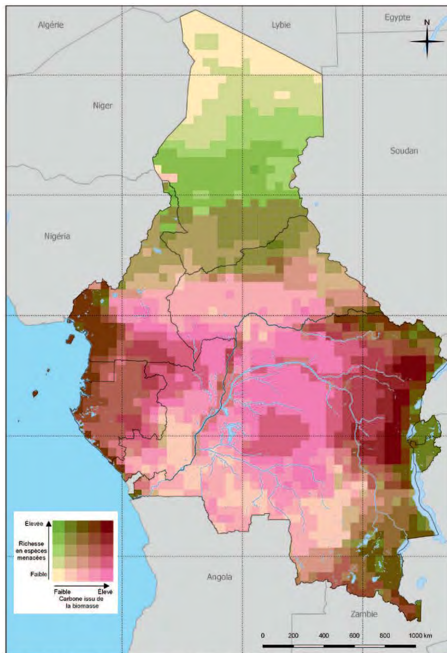
Figure 1.6: Variation spatiale de la densité en carbone et de la richesse spécifique potentielle (espèces menacées)
